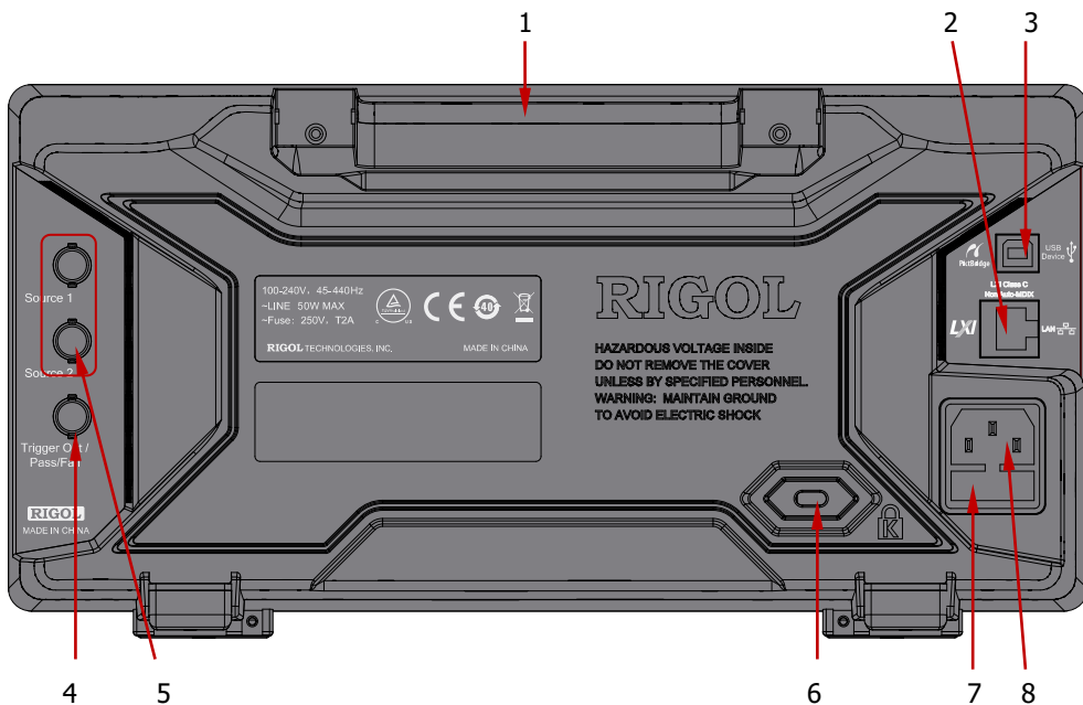
Bild 1- 10 Rückseite Übersicht
