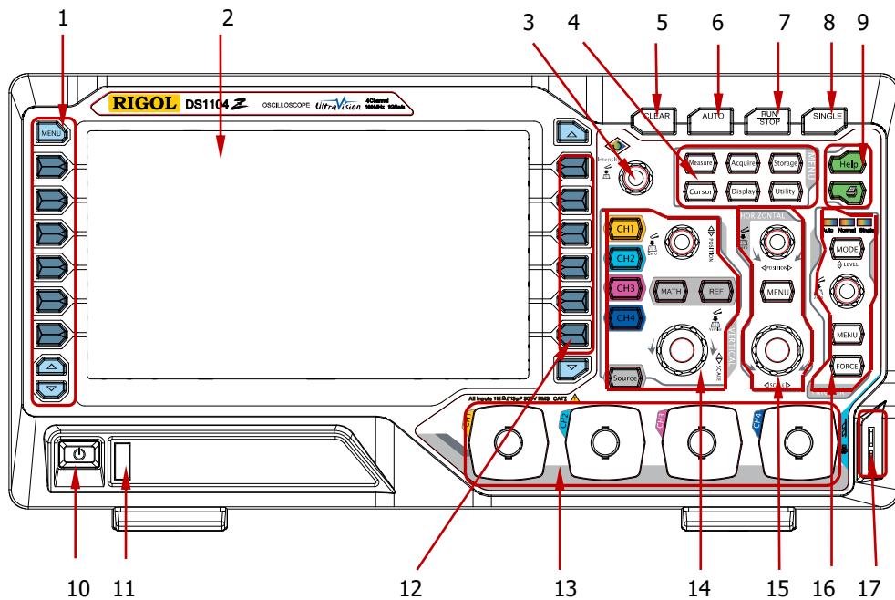
Bild 1-9 Bedienfeld Übersicht
