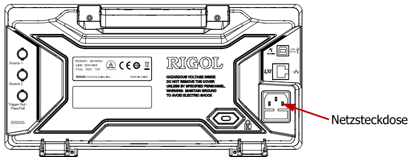
Bild 1-4 Anschluß Stromversorgung
