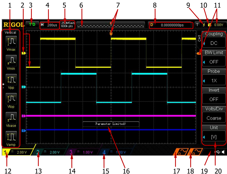
Bild 11 Benutzeroberfläche
