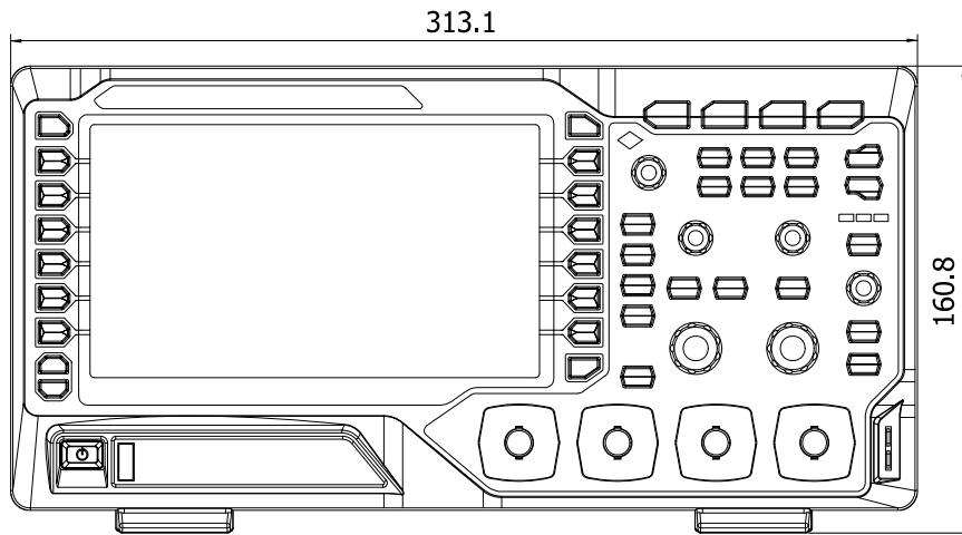
Bild 1-1 Frontansicht
